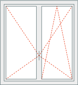
Ouverture à la française, 2 vantaux, avec oscillo-battant
