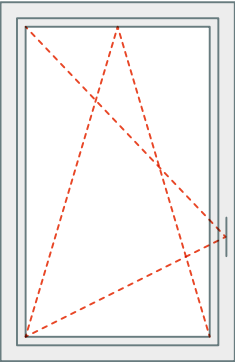
Ouverture à la française, 1 vantail, avec oscillo-battant
