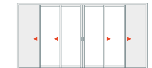
4 VANTAUX / 2 RAILS
